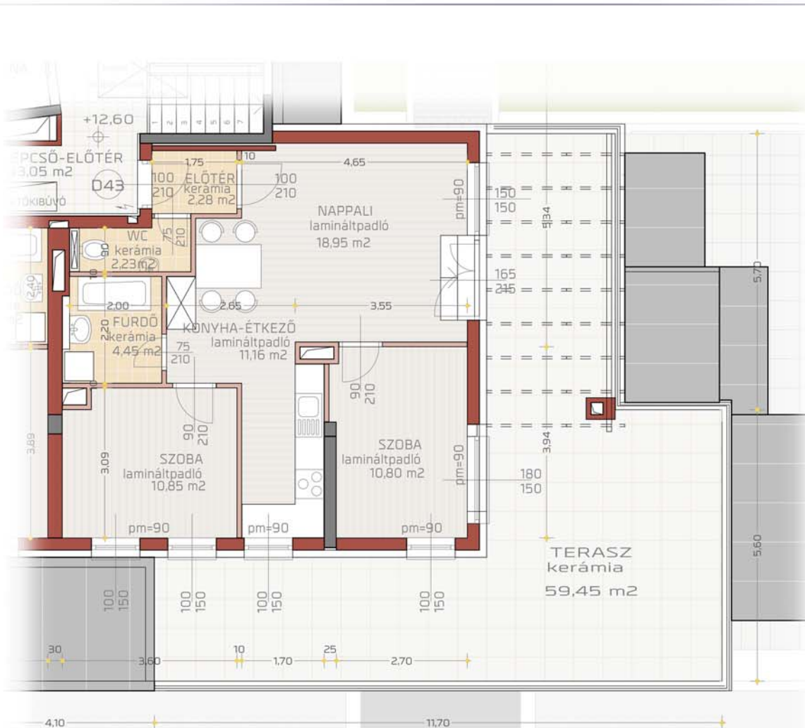
LAKÁS ELHELYEZKEDÉSE
